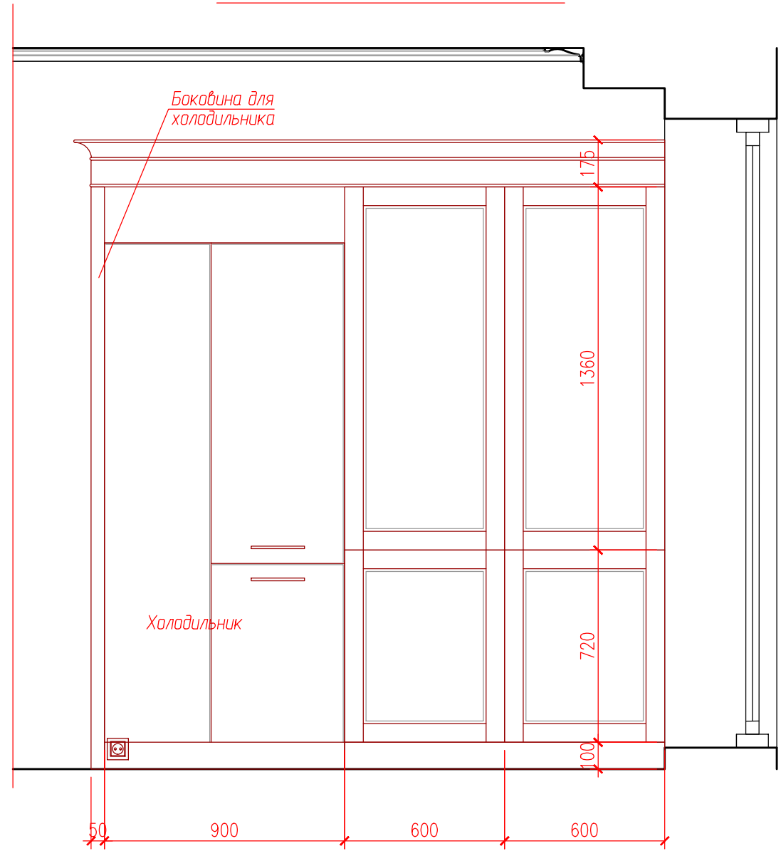
Развертка стен между точками 1-2
