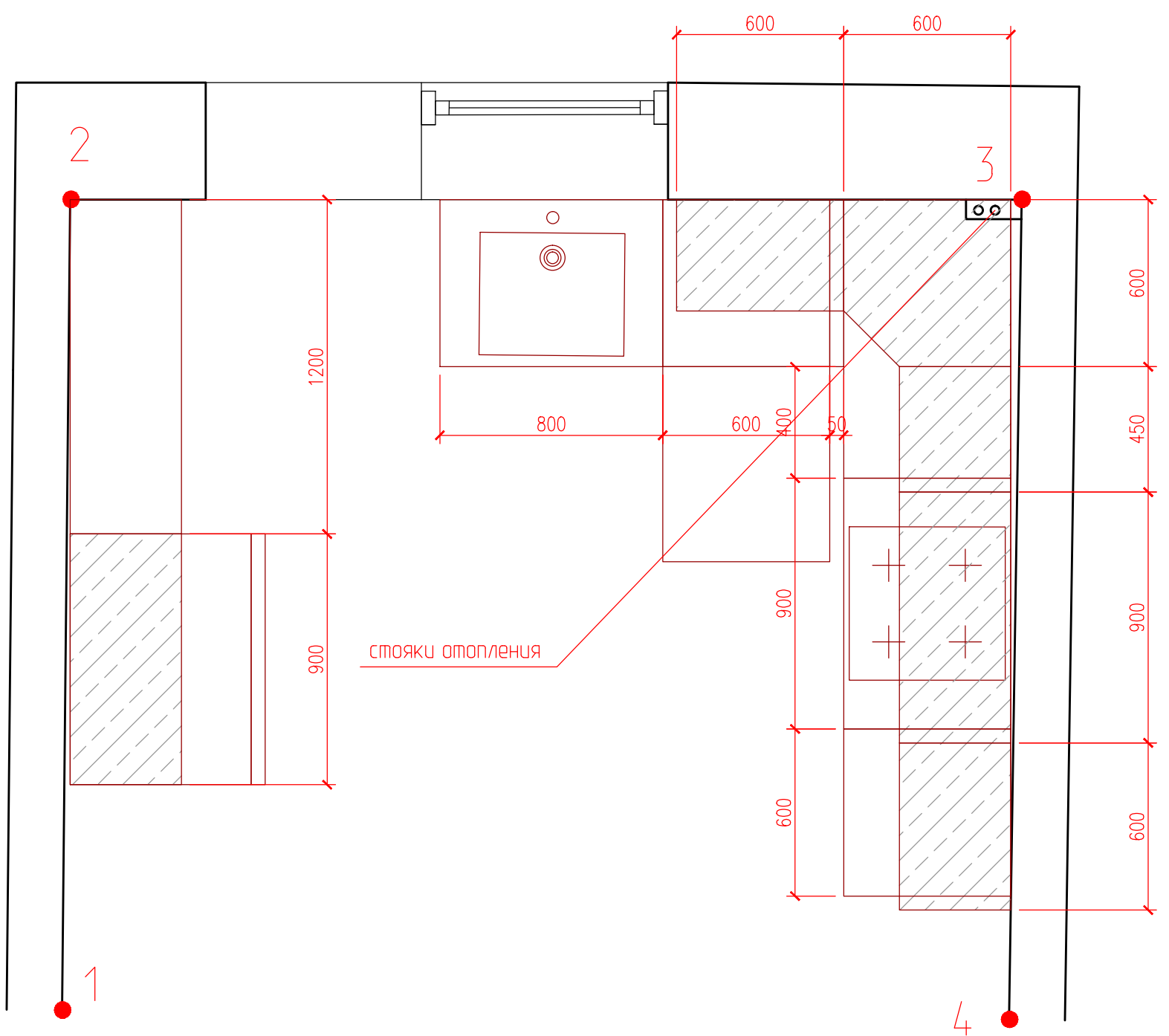
Фрагмент плана кухни
