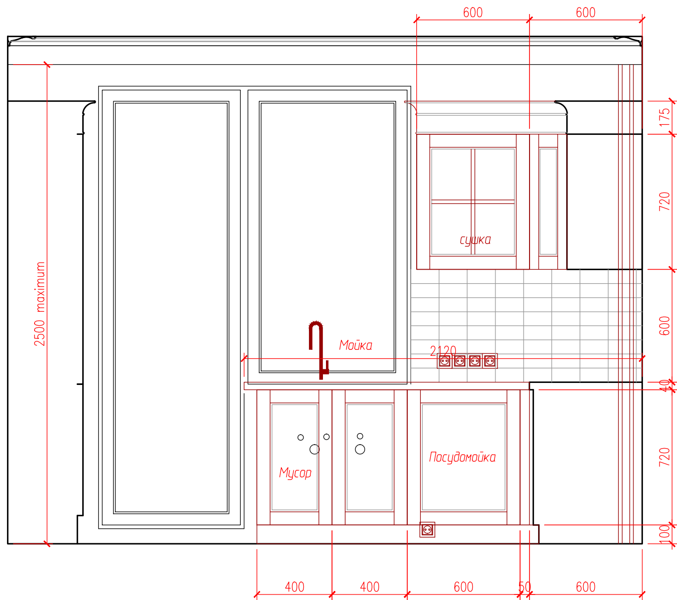
Развертка стен между точками 2-3
