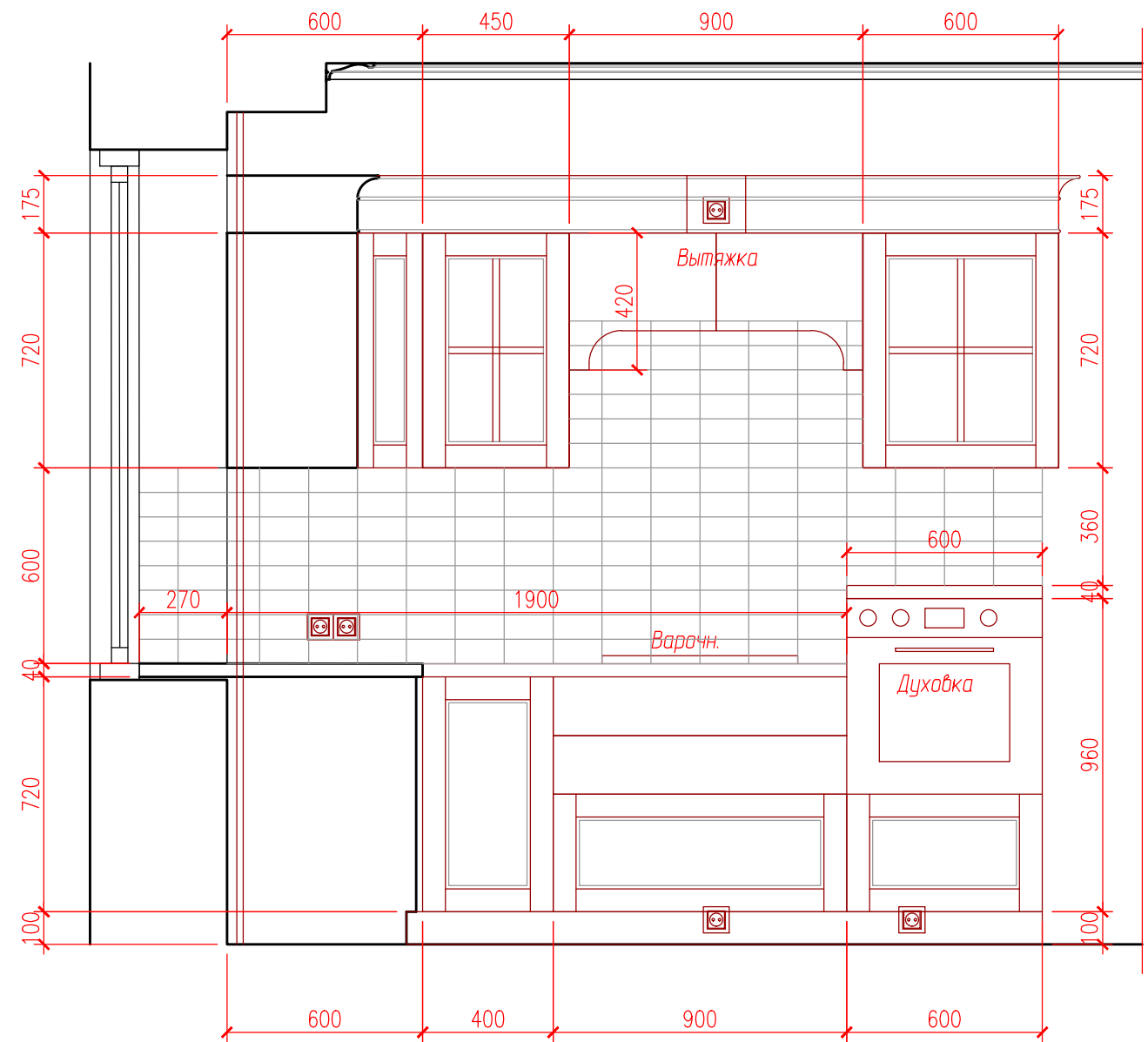
Развертка стен между точками 3-4
